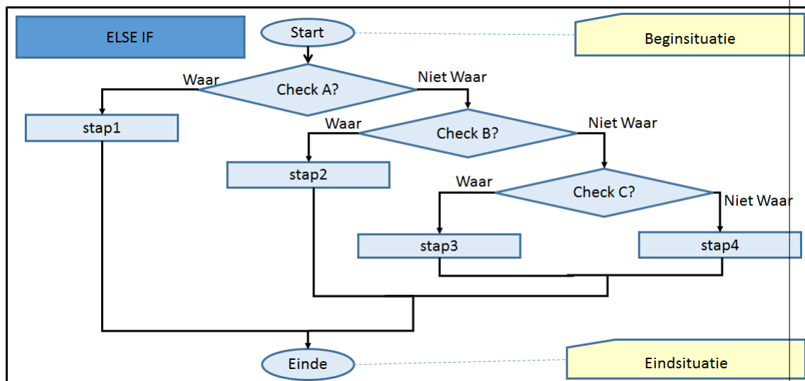
Figuur 1: Stroomdiagram geneste if .. then .. else
